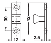
Counterpiece ชิ้นส่วนที่หน้าบาน
