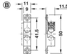
Catch ก้ามปูทองเหลือง
