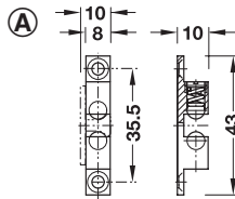
Catch ก้ามปูทองเหลือง
