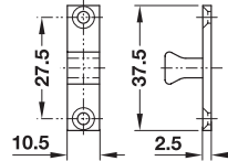
Counterpiece ชิ้นส่วนที่หน้าบาน
